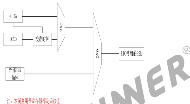
图 6-1: RTC 时钟源
