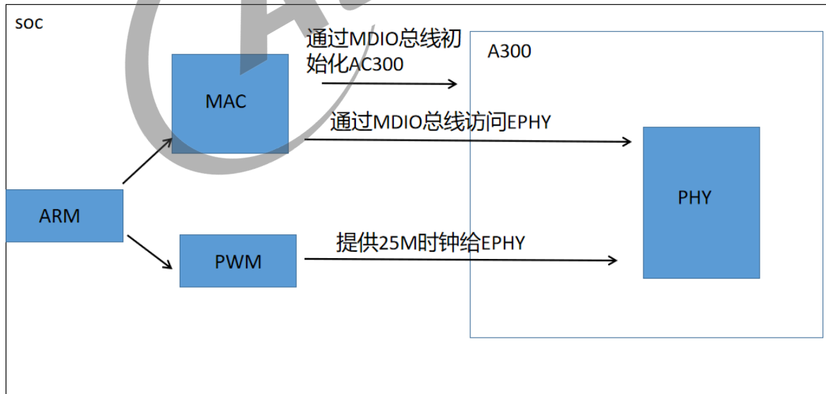
图 3-10: AC300 框图
