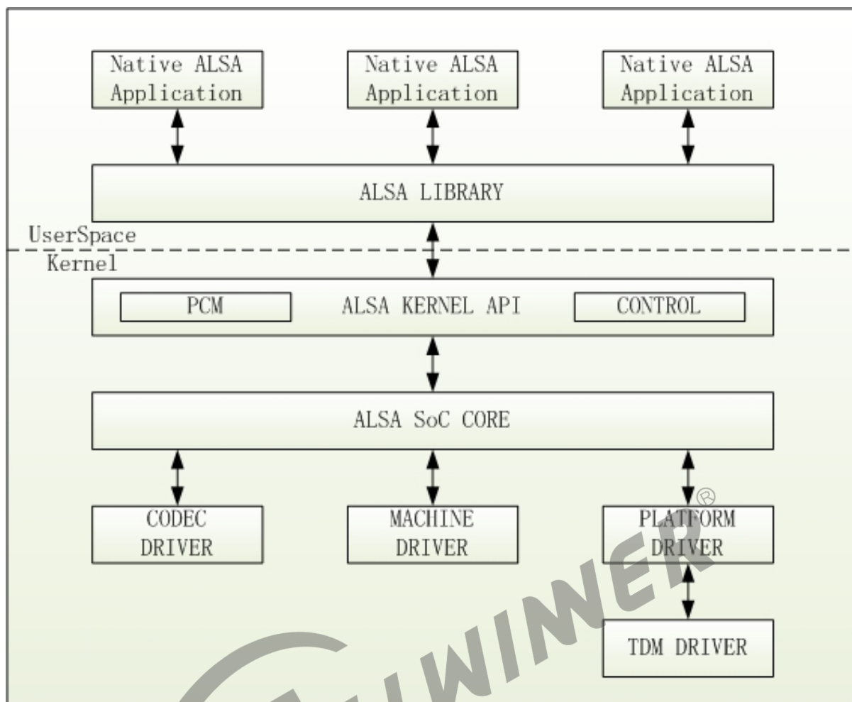
图 2-9: 软件框架图
